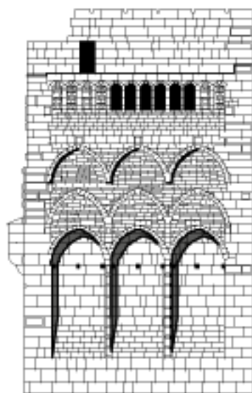
Élévation Nord
