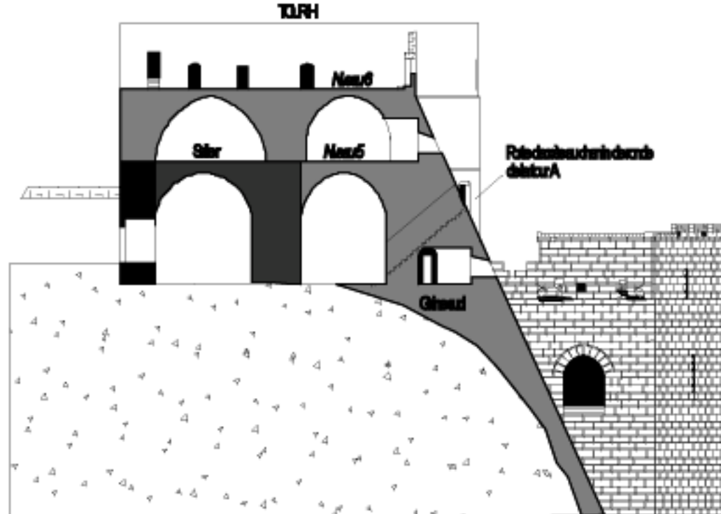
Élévation Ouest de la tour A et coupe sur le "donjon"
