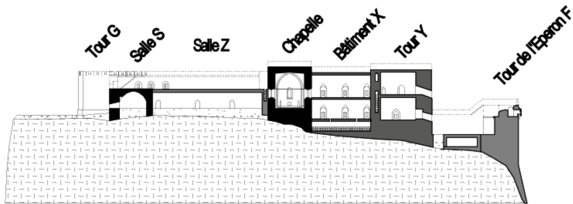
Coupe du château suivant une ligne imaginaire Nord-Sud
