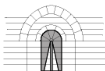
Archère de la tour G Niveau 1
