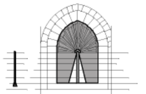
Archère de la tour G Niveau 0
