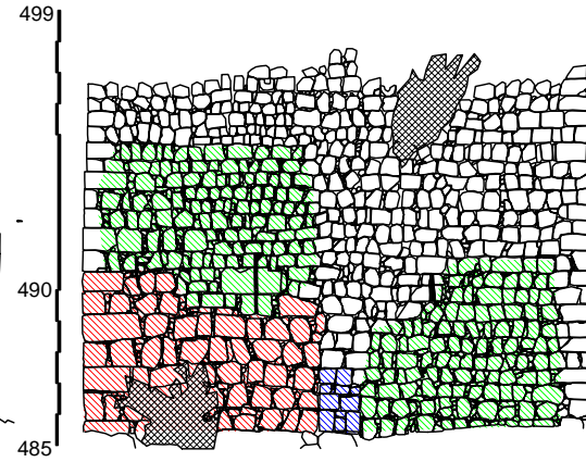
Façade Ouest
