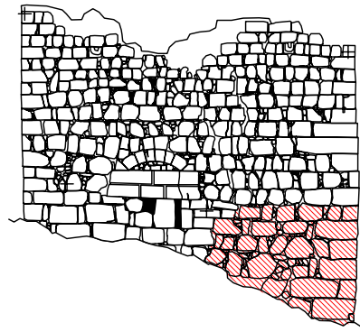
Façade Nord
