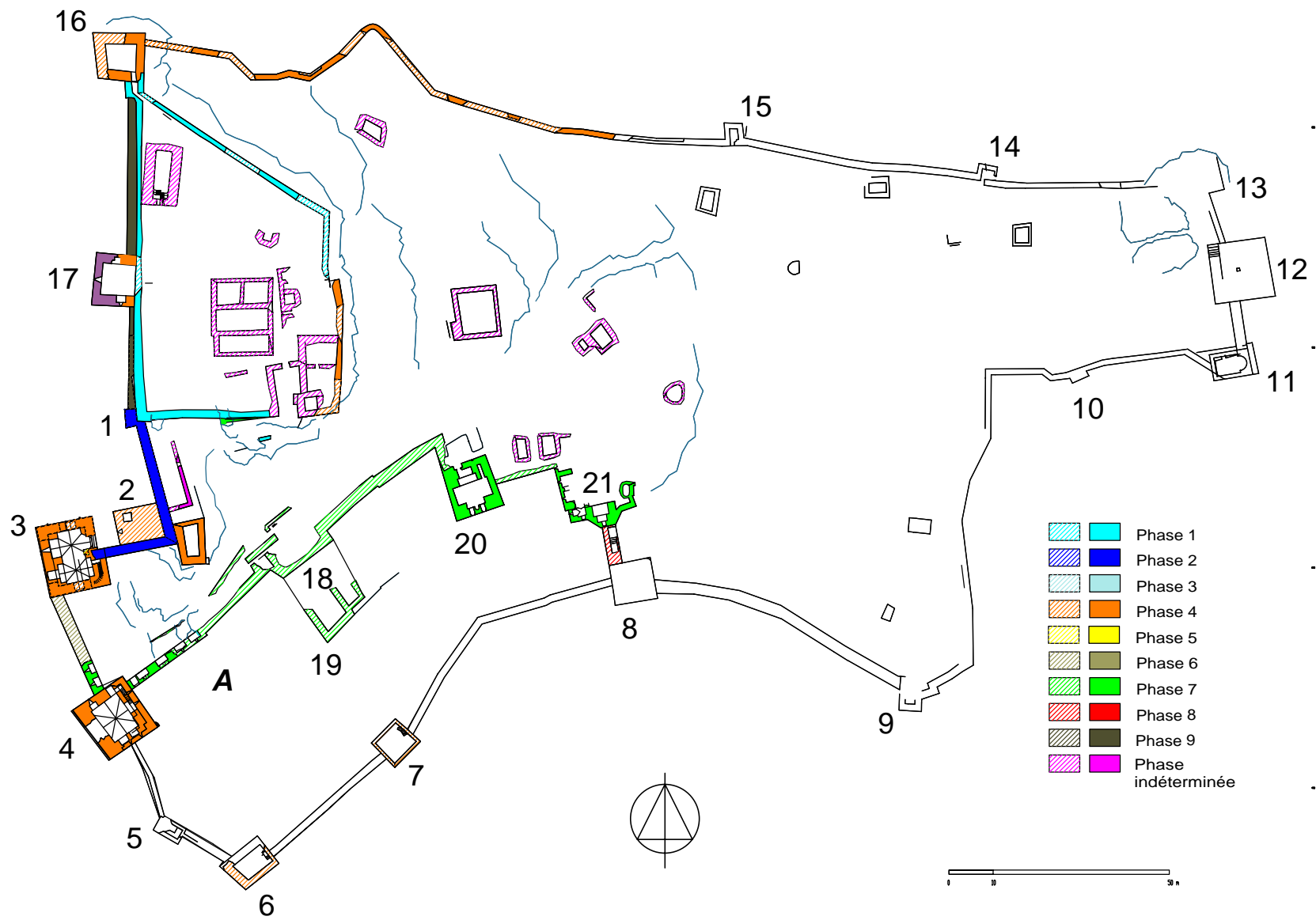
CHATEAU DE BOURZEY - SYRIE PLAN GENERAL - NIVEAU INTERMEDIAIRE Mission Bourzey 2001 J. Mesqui, Ph. Dangles, N. Faucherre, P. Lebel, B. Michaudel
