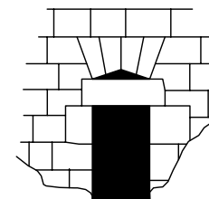
Citerne C1 Élévation de la porte intérieure
