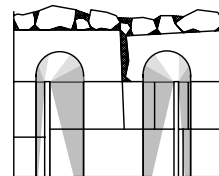
Courtine 1-2. Niveau 0 Archères 7, 8, 9, 10
