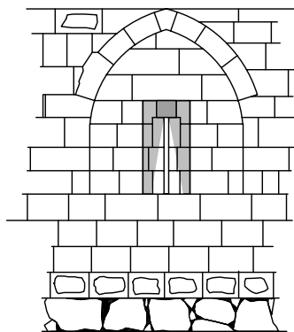
Courtine 2-3. Niveau 1 Archère type
