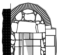
Barbacane de la tour 8 Archère donnant à l'ouest
