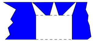
Enceinte extérieure orientale de la ville haute Archère triple
